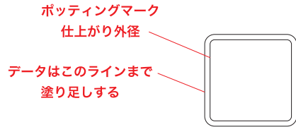
PMS-1 ポットティングマーク仕上がり 15.2×15.2mm データ制作サイズ 17.2×17.2mm
