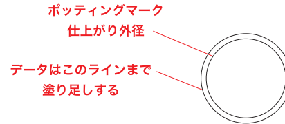
PMS-2 ポットティングマーク仕上がり \phi 15.2mm データ制作サイズ \phi 17.2mm
