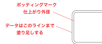
PM-3 ポットティングマーク仕上がり 16.5×16.5mm データ制作サイズ 18.5×18.5mm
