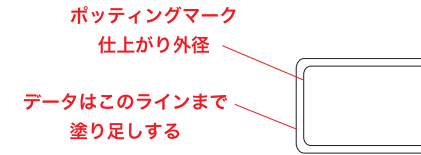
PMS-4 ポットティングマーク仕上がり 10.5×16.5mm データ制作サイズ 12.5×18.5mm
