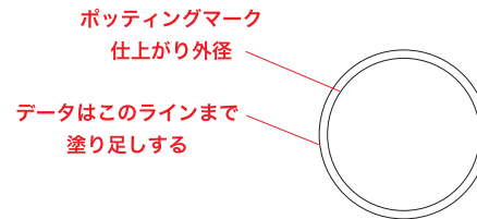
PM-2 ポットティングマーク仕上がり \phi 18.5mm データ制作サイズ \phi 20.5mm
