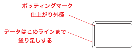
PM-5 ポットティングマーク仕上がり 10.5×16.5mm データ制作サイズ 12.5×18.5mm
